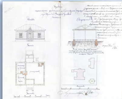
Проект амбулатории для строительства при Сарапульской уездной земской больнице. 1901 г.
