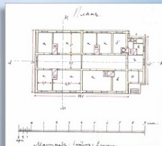
Проект инфекционного барака для строительства в селе Селты Мамыжского уезда Вятской губернии. 1900 г.
